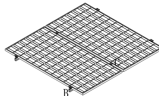
VISTA ISOMÉTRICA
