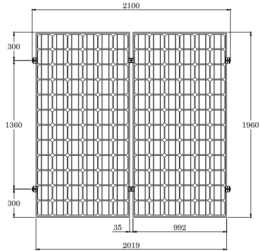
VISTA PLANTA
