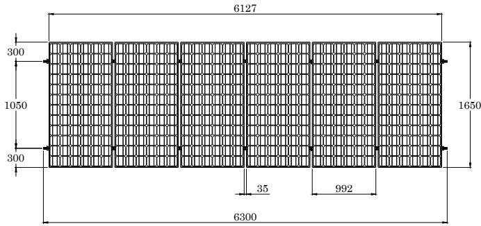
VISTA PLANTA
